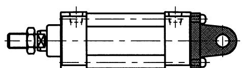
7、CC (单悬耳式)
