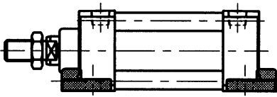
5、FB (后法兰式)
