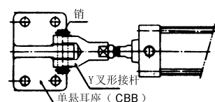
9、杆部叉座式 (RY-CBB)
