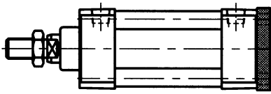
8、CB (双悬耳式)
