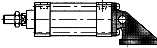
9、CBB (双悬耳座式)
