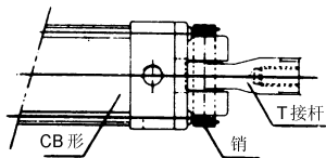
7、双悬耳杆式 (HCB-T)
