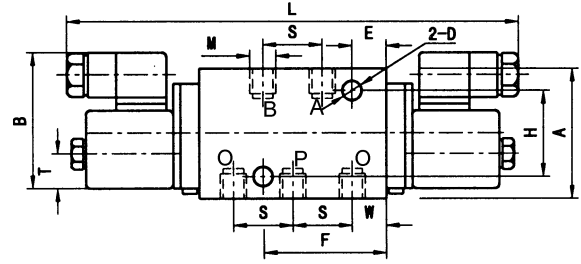
二位五通双电控换向阀
