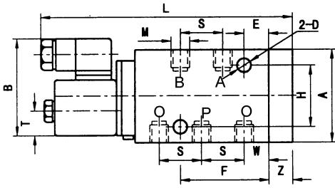
二位五通单电控换向阀
