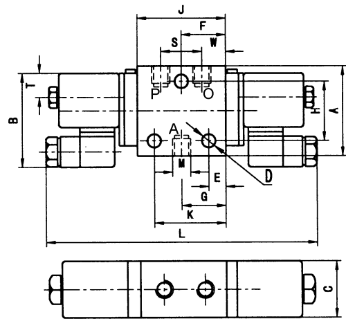
二位三通双电控换向阀
