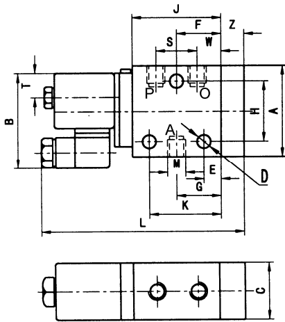
二位三通单电控换向阀
