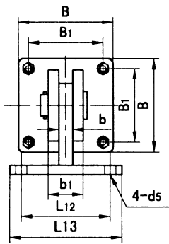
双悬耳座式气缸 (ESZ 型)
