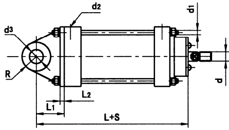
双悬耳式气缸 (ES 型)
