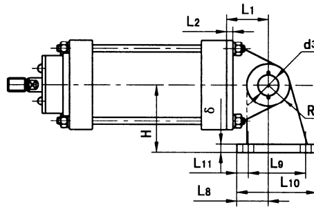
单悬耳座式气缸 (EZ 型)
