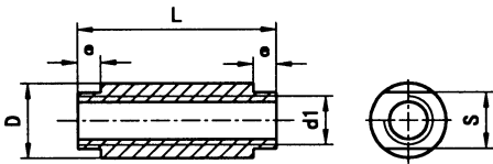
管连接件
