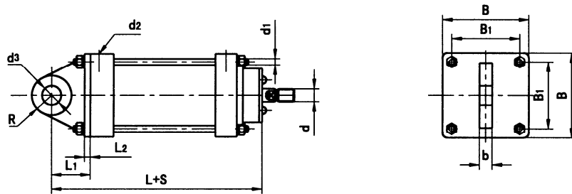
单悬耳式气缸 (E 型)
