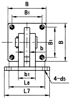
单悬耳座式气缸 (EZ 型)
