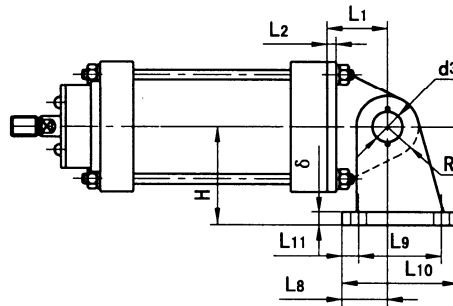
双悬耳座式气缸 (ESZ 型)
