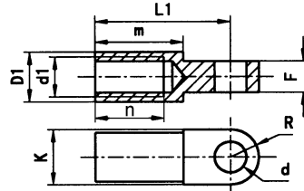
杆连接件
