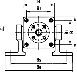
中间铰轴支座式气缸 (ZZ 型)
