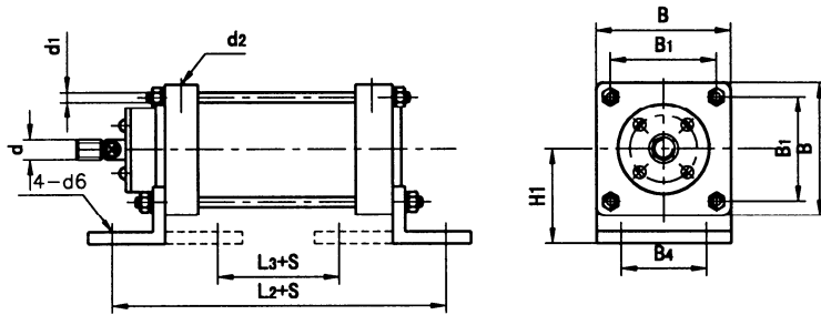
脚架式气缸 (J 型)
