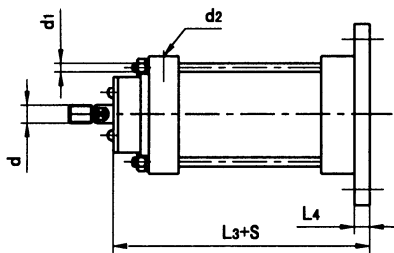
后法兰式气缸 (F 型)
