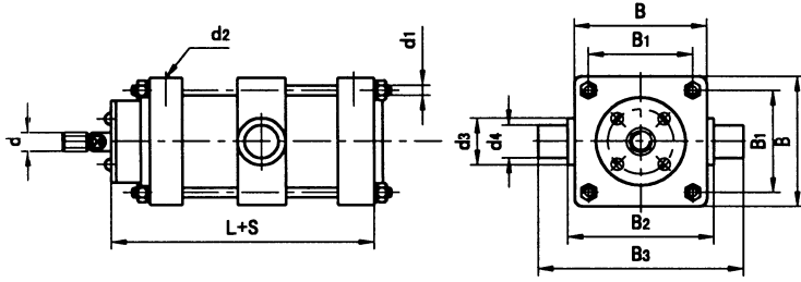
中间铰轴式气缸 (Z 型)
