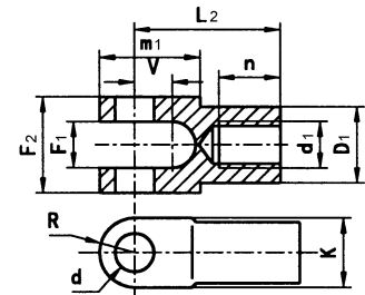
叉连接件
